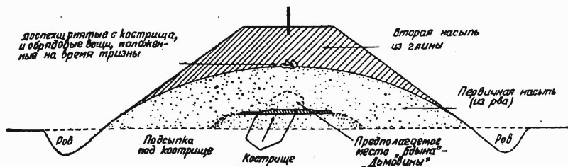
Разрез кургана «Черная Могила» по уточненным данным
