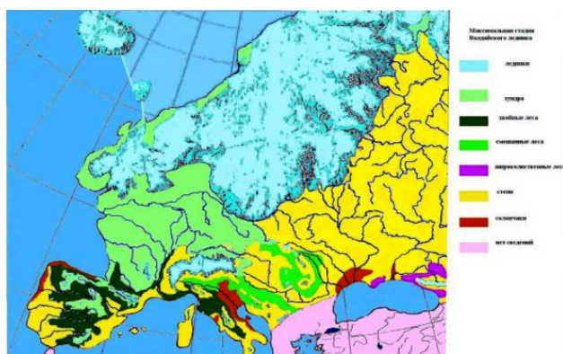
Растительность максимума Валдая
