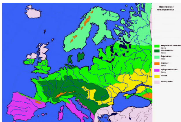
Растительность микулинского межледниковья
